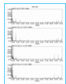
FFT
