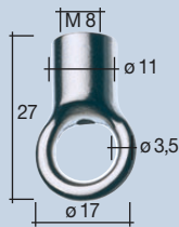
Öse | 5 Eye Œillet
