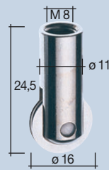
Umlenkrolle | 1 Pulley Poulie de renvoi
