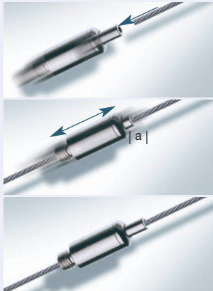
Seilspanner Cable tensioner Tendeur réglable
