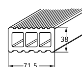
Subframe bar
