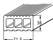
Subframe bar
