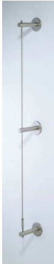
Edelstahlseil 4 mm, 820-0400 einseitig Außengewinde verpresst 850-0400-060 anderseitig Außengewinde verschraubt 826-0400-060 (zur Selbstmontage vor Ort) Stainless steel wire rope 4 mm, 820-0400 one side external thread swaged 850-0400-060 other side external thread swageless connection 826-0400-060 (for self assembly on site)
