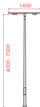
COLUMNA UMA DOBLE
