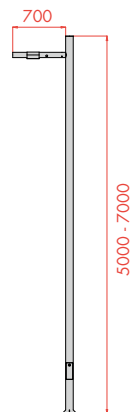
COLUMNA UMA CILÍNDRICA
